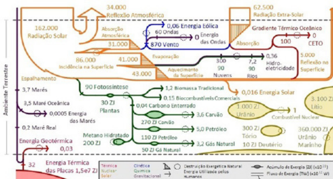
Figura 1. Fluxograma da energia, armazenamento e distribuição
